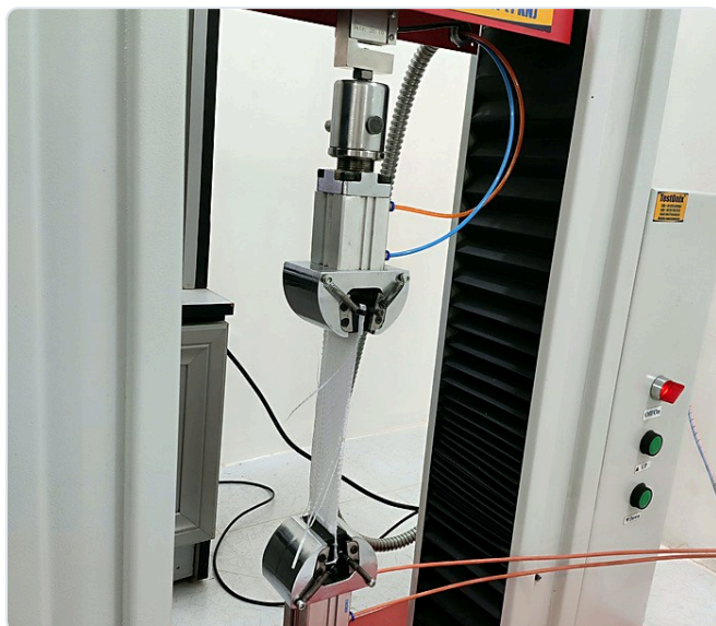
Испытание ткани на разрыв — лаборатория фабрики-партнёра
