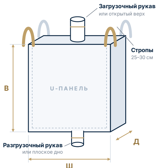
Конструкция: верх, дно, стропы и размеры — под заказ
